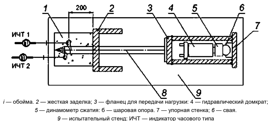
Рисунок Б.1 — Испытание сваи выдергивающей нагрузкой
