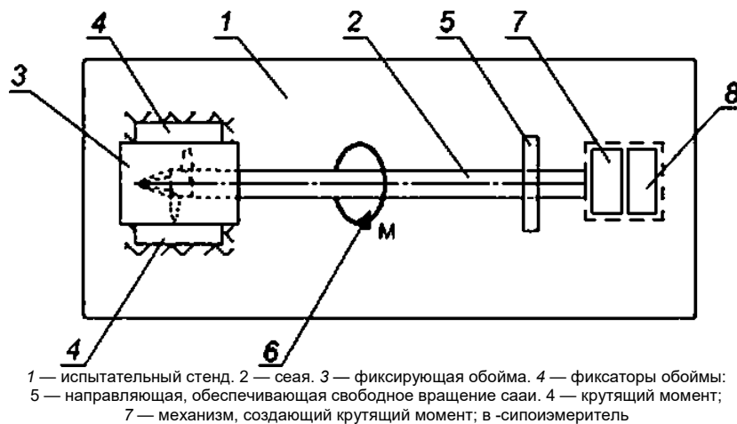
Рисунок Б.2 — Схема испытания сваи крутящим моментом
